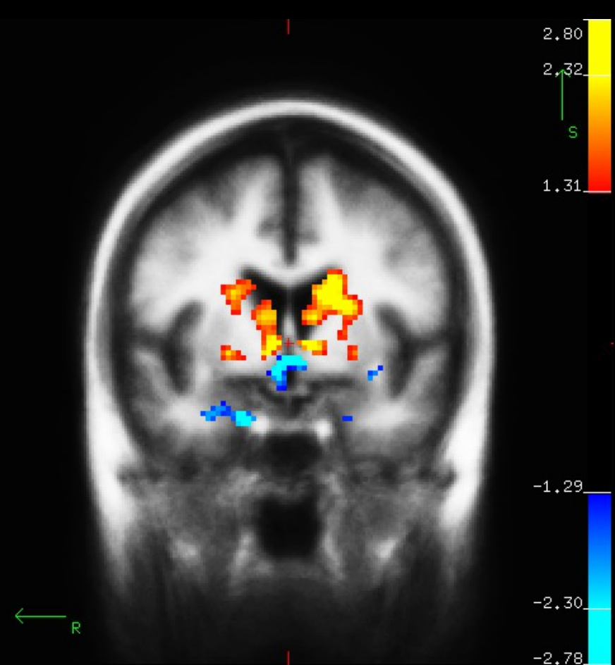
Mni305 Space
